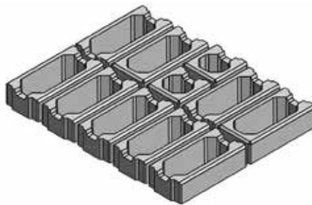
Paredo ® Trend Versandereinheit: 1 Lage (0,4 m 2 ) bestehend aus 7 x Grundstein (40 x 20 x 10 cm), 2 x Endstein (40 x 20 x 10 cm) und 2 x Halbendstein (20 x 20 x 10 cm)
