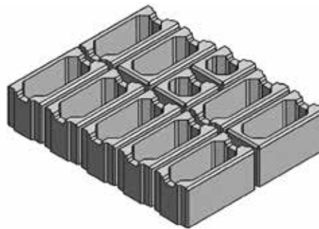
Paredo Basic Versandereinheit: 1 Lage (0,8 m 2 ) bestehend aus 7 x Grundstein (40 x 20 x 20 cm), 2 x Endstein (40 x 20 x 20 cm) und 2 x Halbendstein (20 x 20 x 20 cm)
